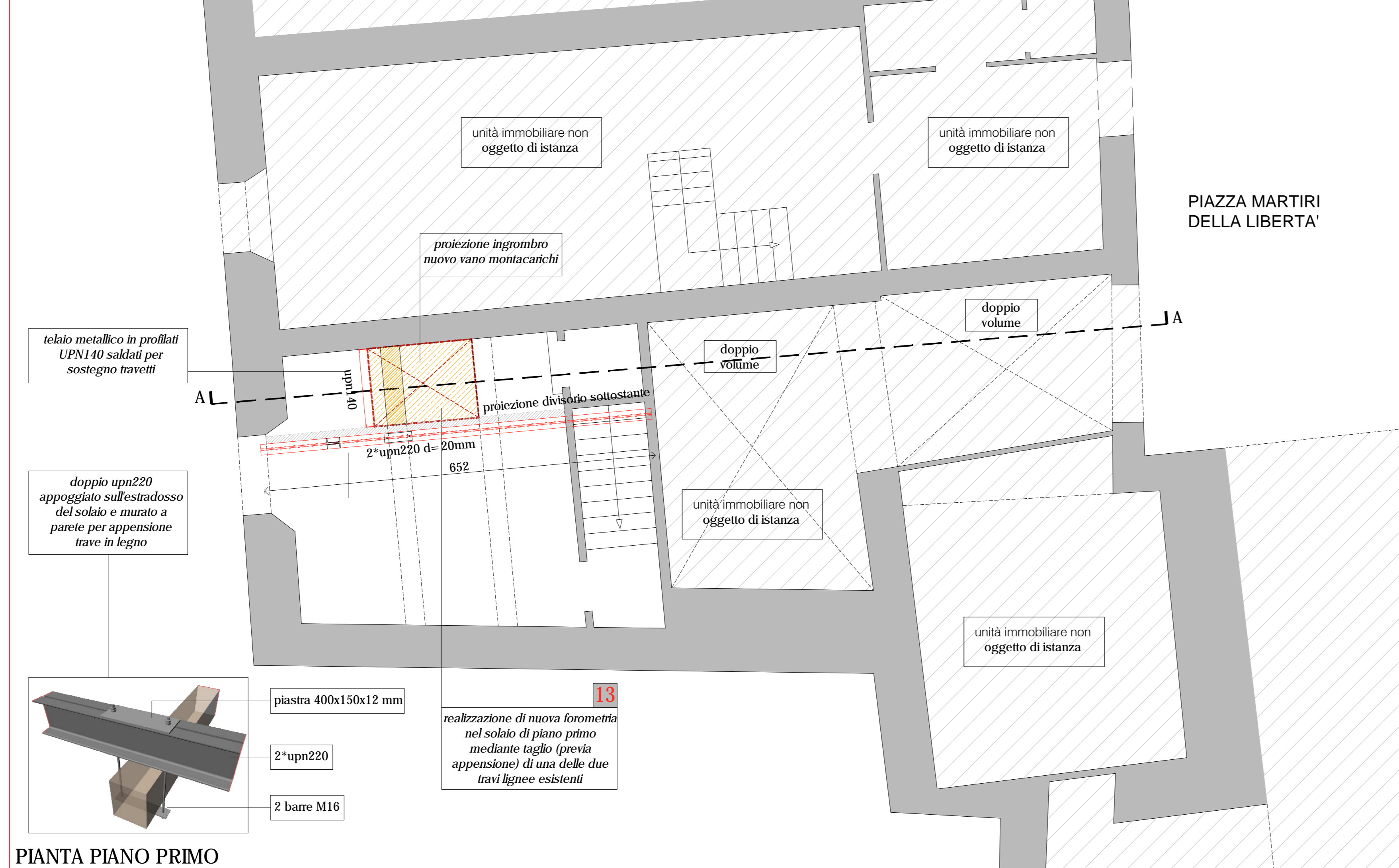
PIANTA PIANO PRIMO
