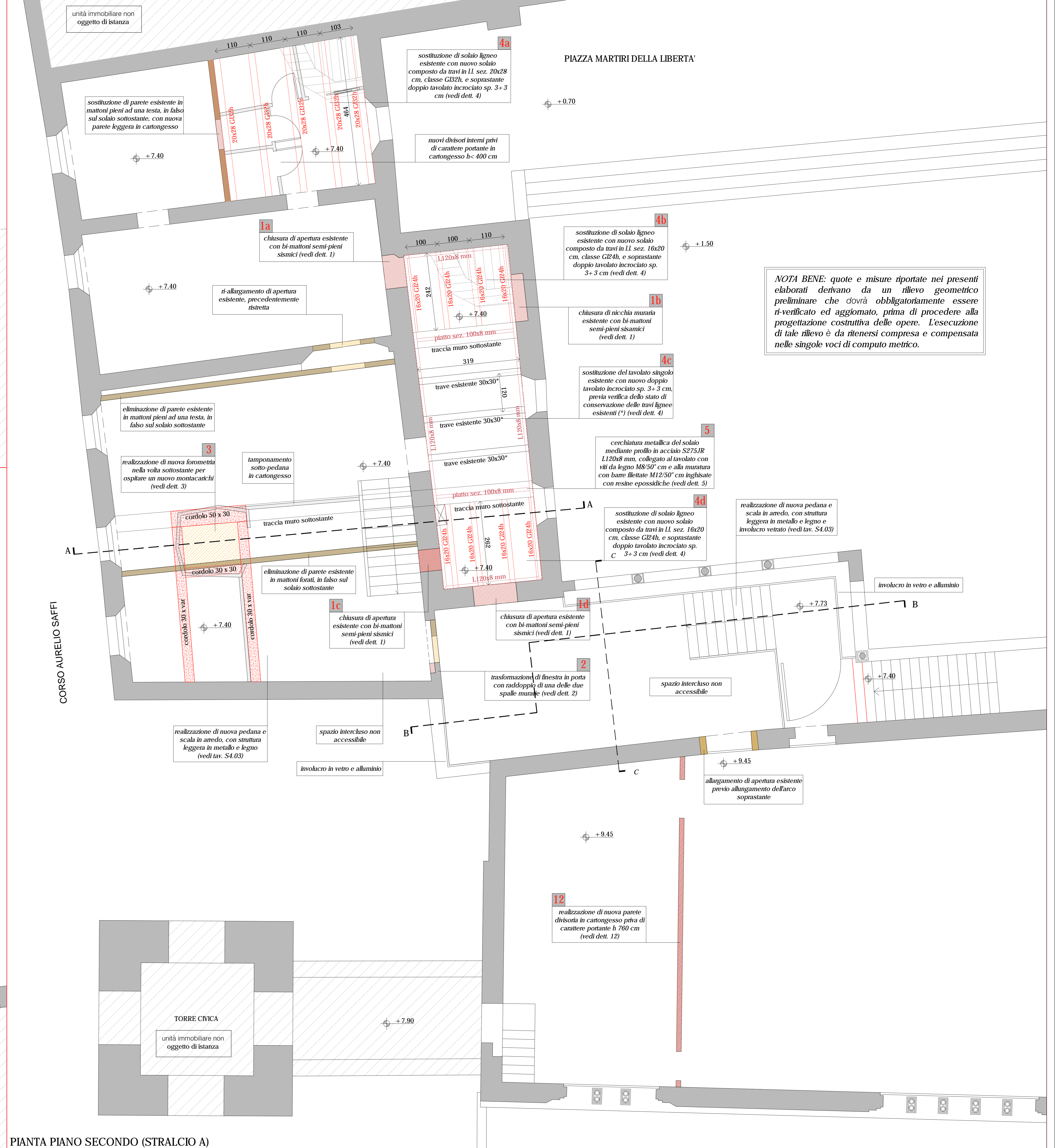
PIANTA PIANO SECONDO (STRALCIO A)
